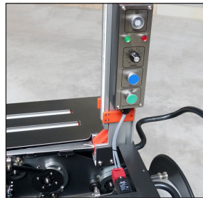
Alle Einstellungen bequem von außen am Bedienfeld
