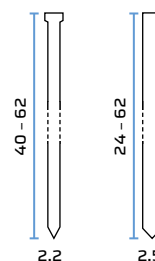
Senkkopfstift Typ SK 500/ Stift S 500 Brad Type SK500 Pin Type S 500
