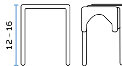
KS 123 und Heftklammer Typ 95 KS 123 and staple type 95
