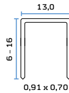
Klammer Typ 80/380 Staple Type 80/380
