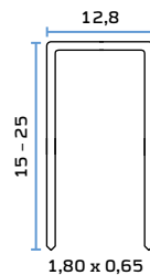
Klammer Typ 110 Staple Type 110
