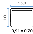
Klammer Typ 80/380 Staple Type 80/380
