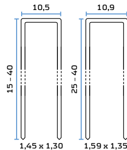
Klammer Typ 14 + 16 (155) Staple Type 14 + 16 (155)
