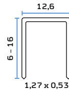
Klammer Typ 95 Staple Type 95
