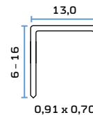
Klammer Typ 80/380 Staple Type 80/380
