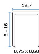
Klammer Typ 72 Staple Type 72
