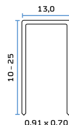
Klammer Typ 80/380 Staple Type 80/380
