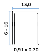
Klammer Typ 80/380 Staple Type 80/380
