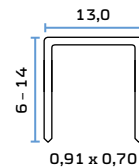
Klammer Typ 80/380 Staple Type 80/380
